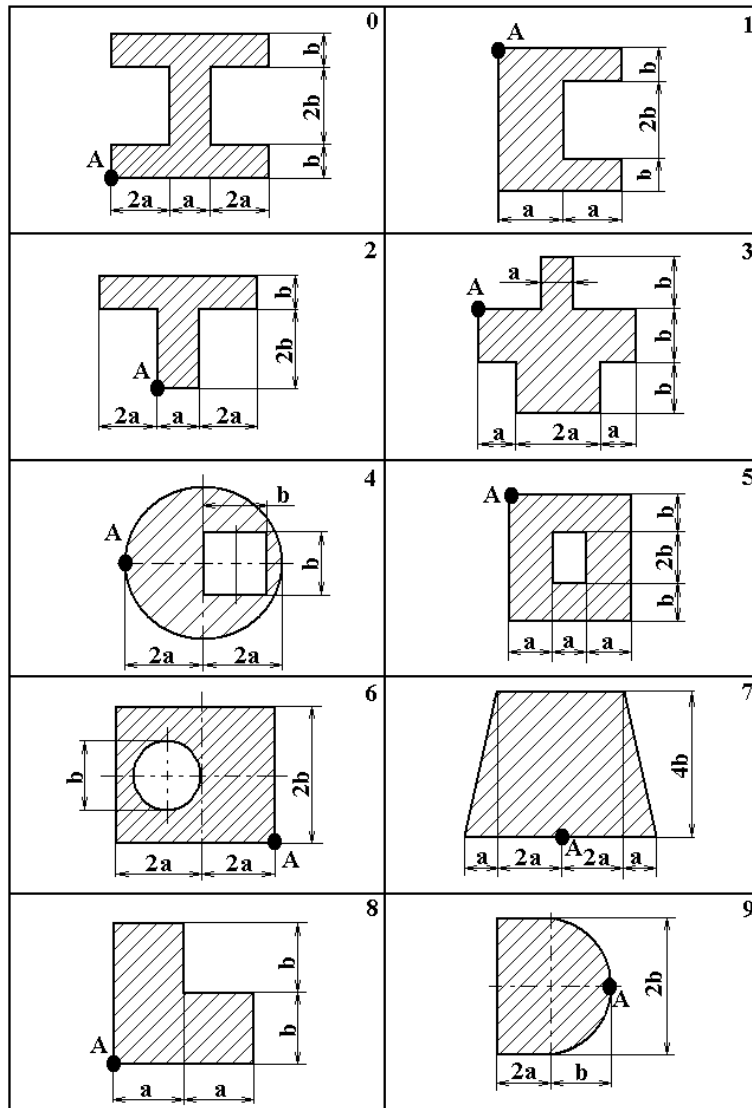
Рисунок 5.1 – Схемы сечений
