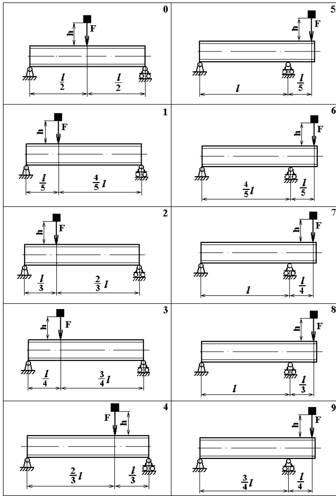
Рисунок 8.2 – Схемы нагрузки на балку
