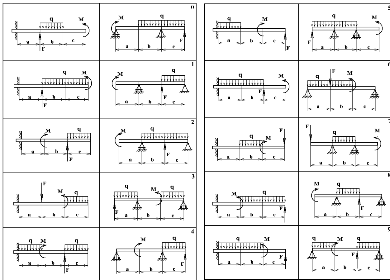
Рисунок 4.1 – Схемы балок и нагрузки
