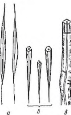
Рис. 1.2 – Продольный вид и поперечный срез элементарного льняного волокна
