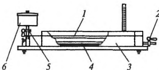
Рис. 12.1. Схема прибора ПДС для определения светостойкости текстильных материалов: 1 – стальные трубки; 2 – кран для слива раствора; 3 – стальная ванна; 4 – люминесцентные лампы; 5 – кран для подачи раствора; 6 – сосуд
