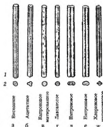
Рис. 1.5 – Продольный вид и поперечный срез искусственных волокон: а) вискозное, б) ацетатное, в) капроновое, г) лавсановое, д) нитроновое, е) нитроновое, ж) хлориновое
