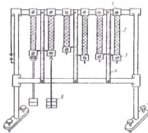
Рис. 5.1. Схема релаксометра типа «стойка» для испытаний материалов при постоянной нагрузке: 1, 3 – зажимы, 2 – проба, 4 – шкала, 5 – штурвальное колесо, 6 – груз
