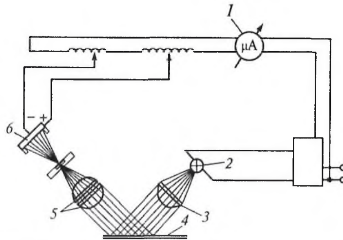
Рис. 10.1. Схема фотоэлектрического блескометра ФБ-2: 1 – микроамперметр; 2 – фотоэлемент; 3, 5 – линзы; 4 – исследуемая поверхность; 6 – источник света
