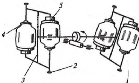
Рис. 13.1. Схема прибора для химической чистки в лабораторных условиях: 1 – банка; 2 – стопорный винт; 3 – крестовина; 4 – подвижная чашка; 5 – неподвижная чашка
