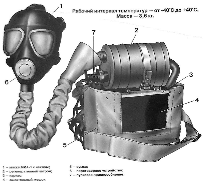
Рис. 12. Противогаз ИП-4М с маской МИА-1.
