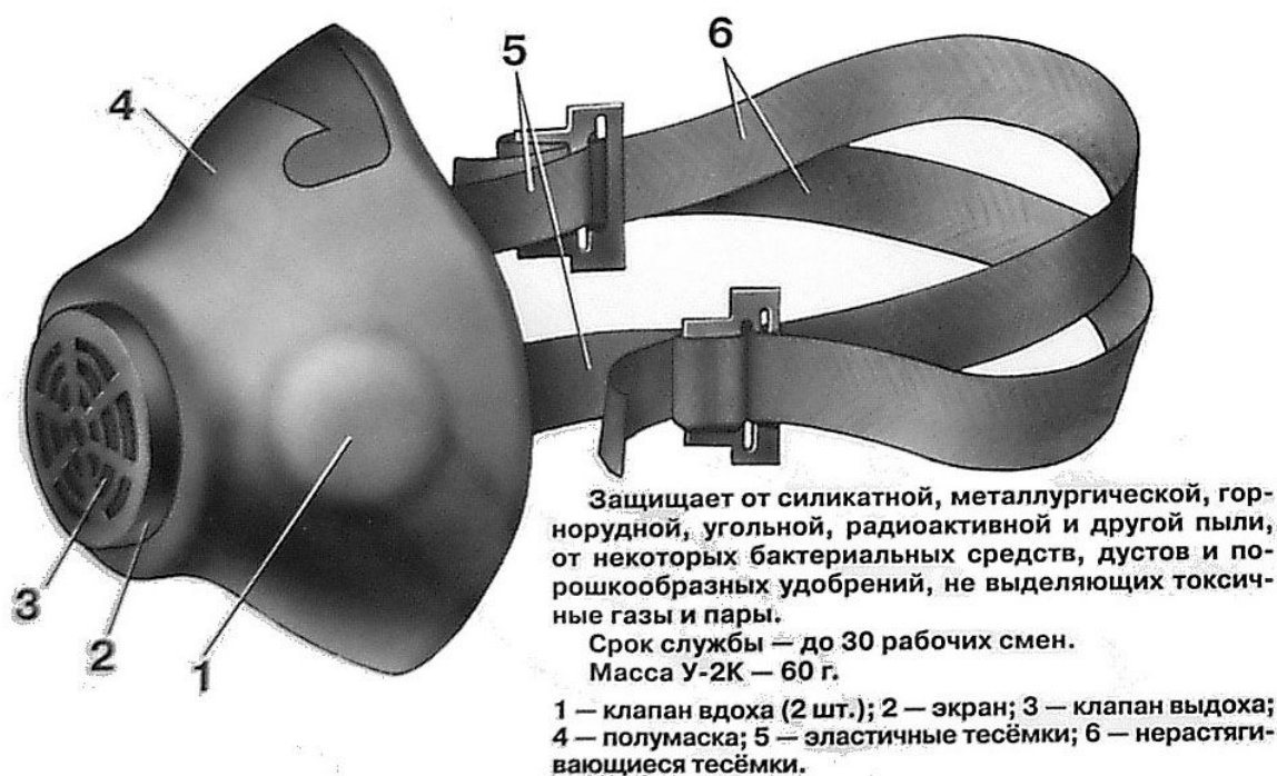
Рис. 22. Респиратор противопылевой У-2К (Р-2).
