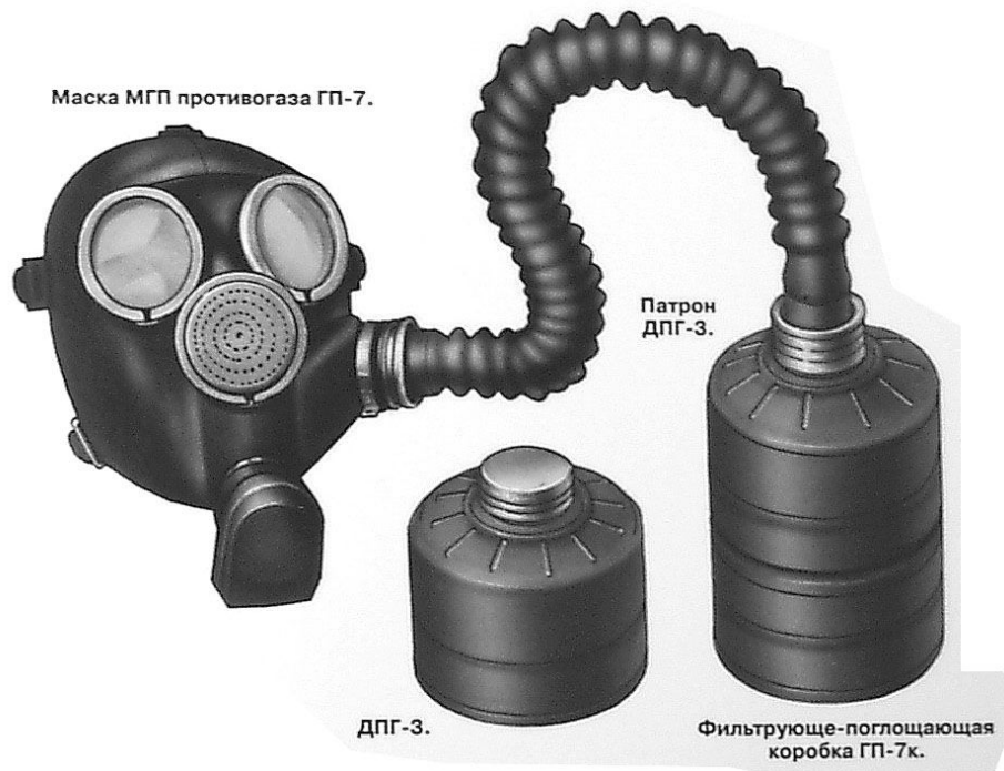
Рис. 9. Дополнительный патрон ДПГ-3.
