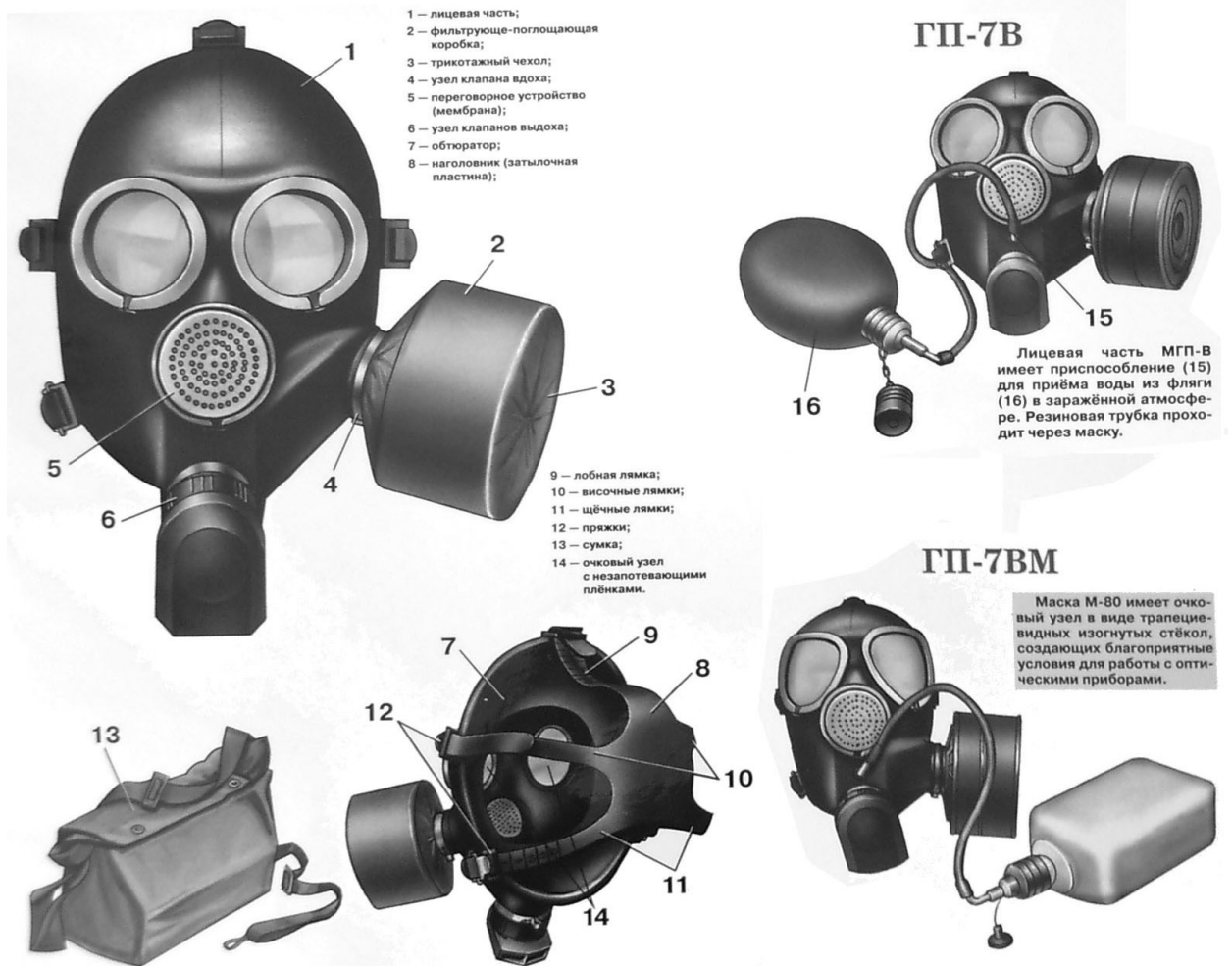
Рис. 6. Противогаз ГП – 7 и его модификации.
