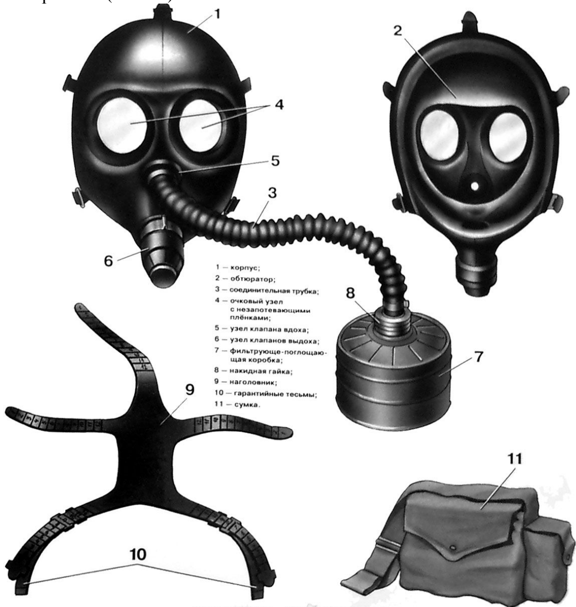
Рис. 7. Противогаз детский фильтрующий ПДФ-7.
