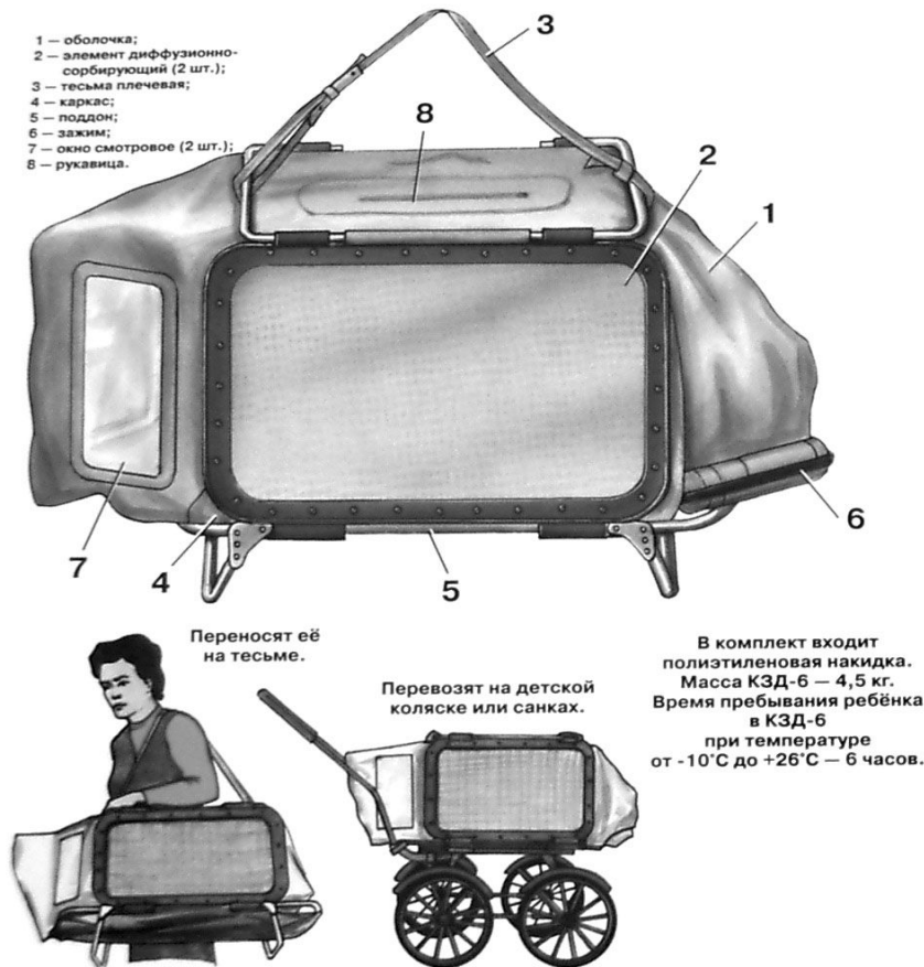
Рис. 8. Камера защитная детская.
