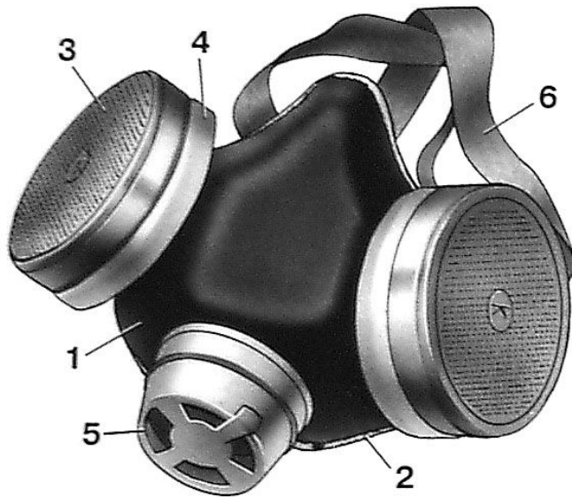
1 — резиновая полумаска; 2 — обтюратор; 3 — поглощающий патрон, 3а — фильтрующе- поглощающий патрон; 4 — пластмассовые манжеты с клапанами вдоха; 5 — клапан выдоха с предохранительным экраном; 6 — оголовье.
