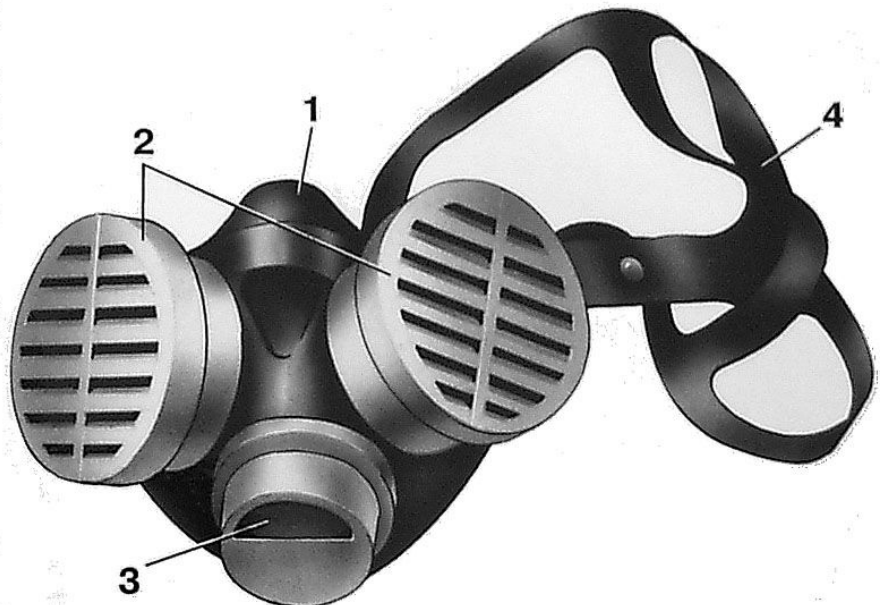
Рис. 25. Респиратор противопылевой РПА-1
