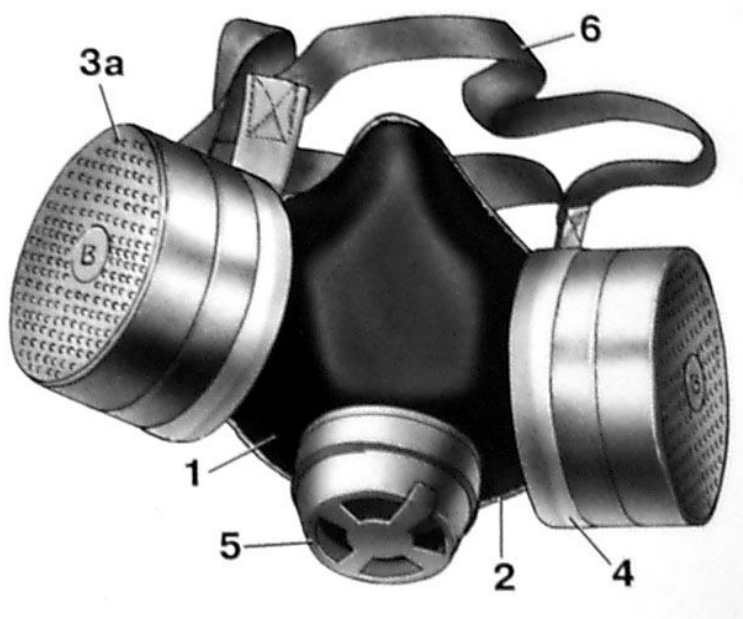
1 — резиновая полумаска; 2 — обтюратор; 3 — поглощающий патрон, 3а — фильтрующе- поглощающий патрон; 4 — пластмассовые манжеты с клапанами вдоха; 5 — клапан выдоха с предохранительным экраном; 6 — оголовье.
