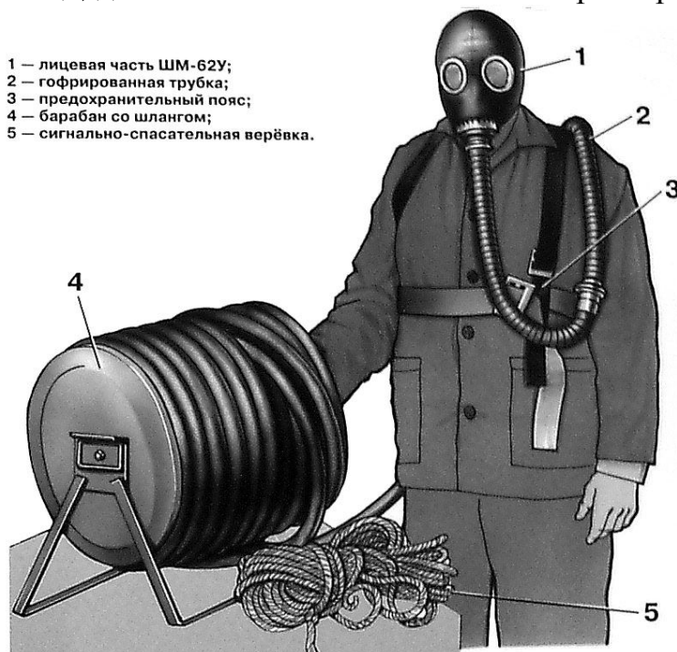
Рис. 18. Противогаз шланговый ПШ-1Б.
