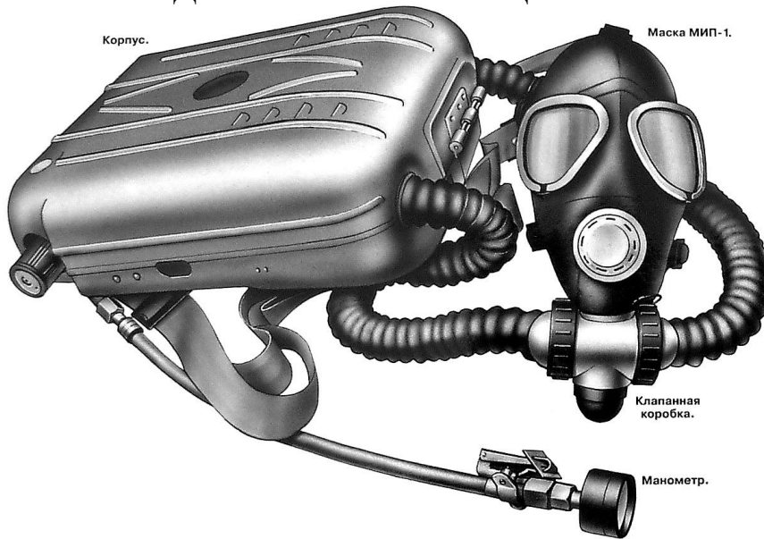
Рис. 13. Противогаз КИП-8.
