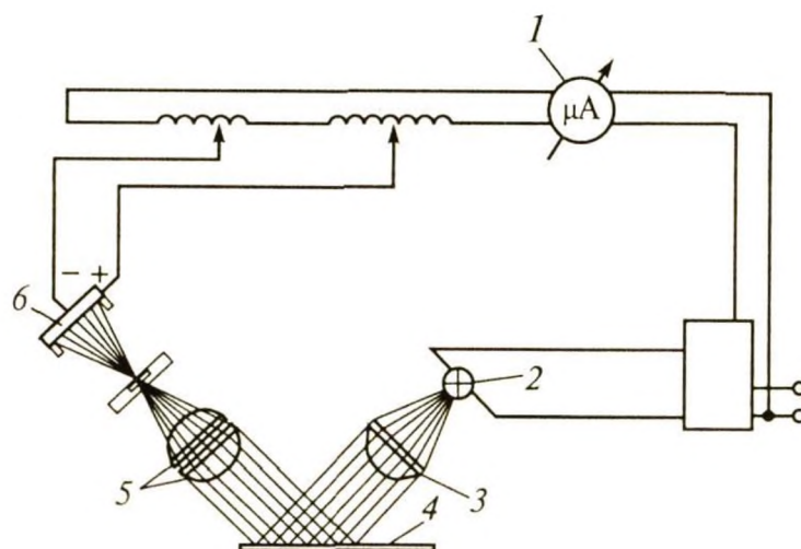
Рис. 10.1. Схема фотоэлектрического блескометра ФБ-2: 1 – микроамперметр; 2 – фотоэлемент; 3 – линзы; 4 – исследуемая поверхность; 6 – источник света
